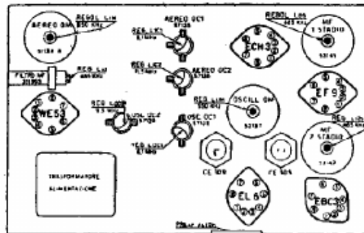
Telaio visto di sotto.
