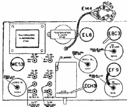
Telaio visto di sopra
