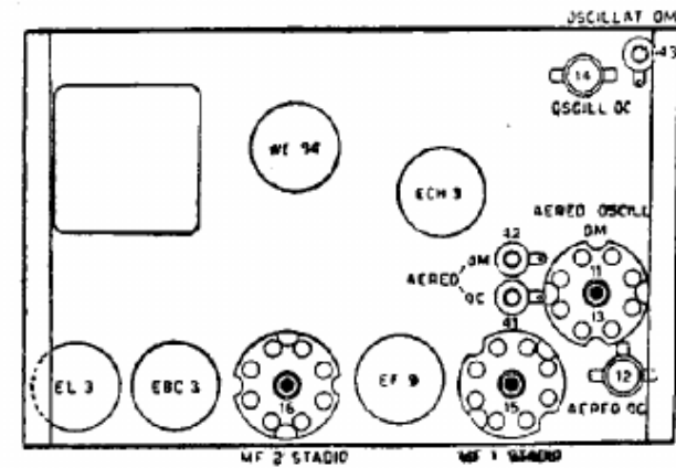
Mod. 580 - Telaio visto di sotto.
